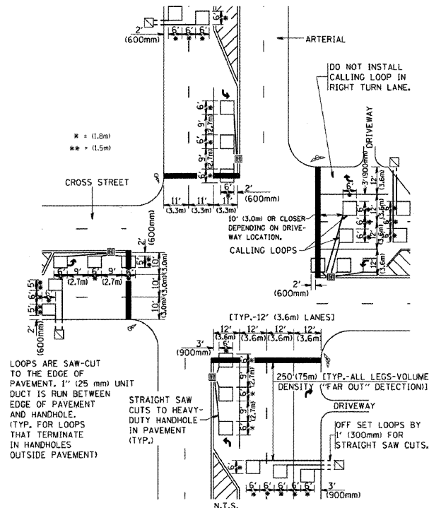
DETAIL 1 N.T.S.
