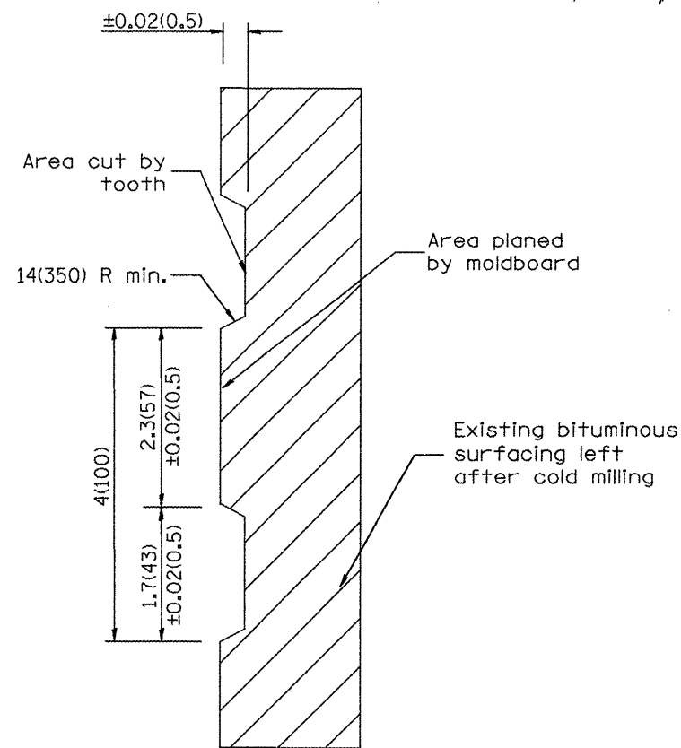
SECTION A-A
