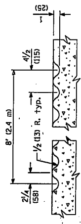
SECTION D-D
