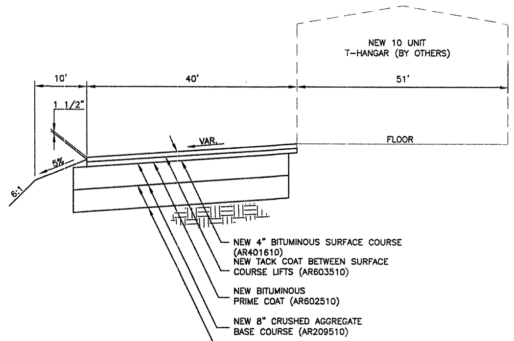
T-HANGAR AND APRON SECTION C-C N.T.S.
