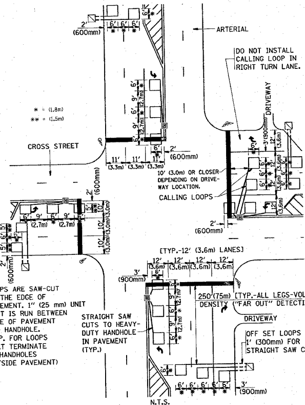
DETAIL 1 N.T.S.
