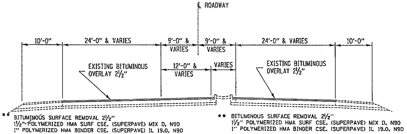
TYPICAL SECTION ④ IL ROUTE 17 STA. 303+00 TO STA. 313+97
