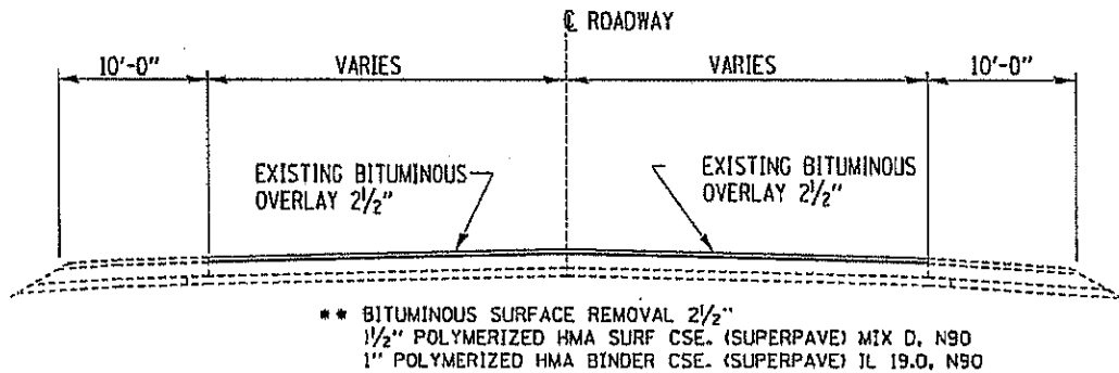
TYPICAL SECTION ⑤ IL ROUTE 17 STA. 313+97 TO STA. 317+76
