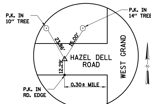
RAMPD PC1, SET P.K. NAIL STA. 44+04.35 @ RAMP D
