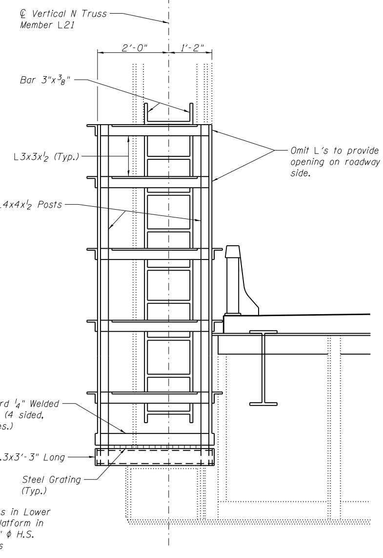
VIEW A-A
