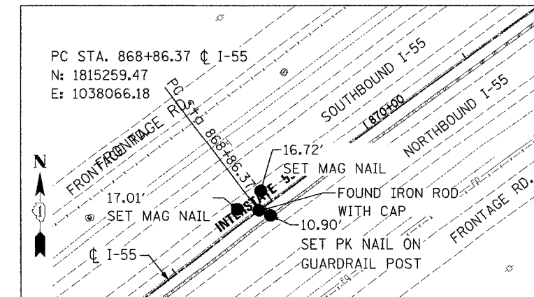
PC STA. 868+86.37
