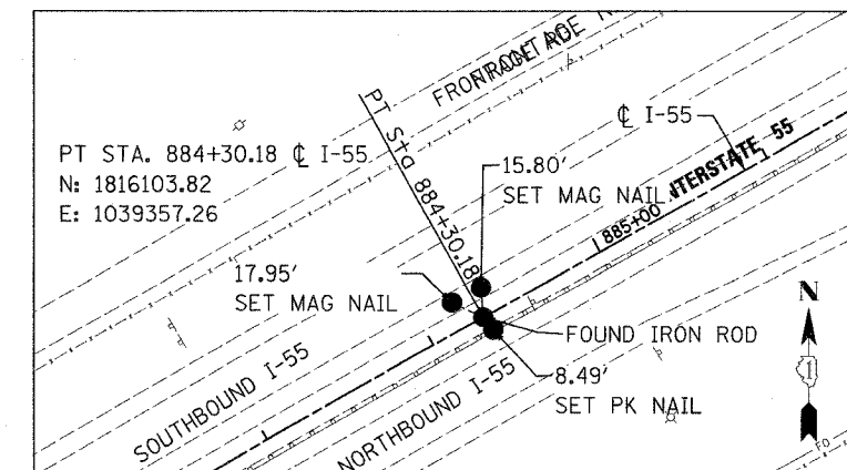
PT STA. 884+30.18
