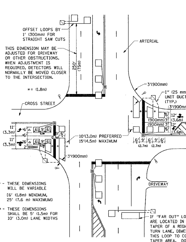
DETAIL 2 N.T.S.
