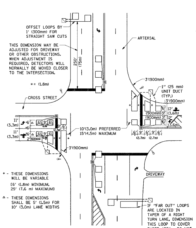
DETAIL 2 N.T.S.
