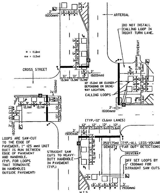
DETAIL 1 N.T.S.
