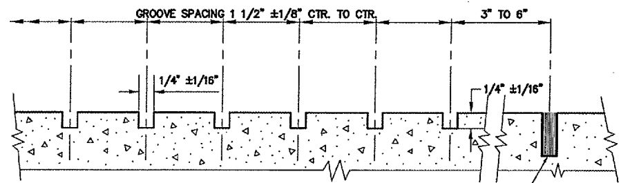
GROOVE DIMENSIONS N.T.S.
