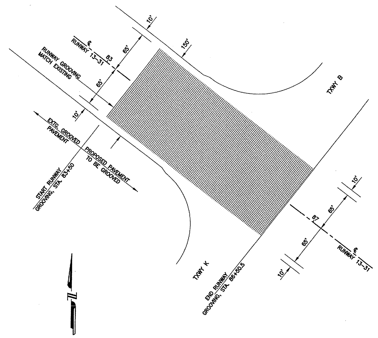
GROOVING PLAN
