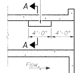
LONGITUDINAL SECTION
