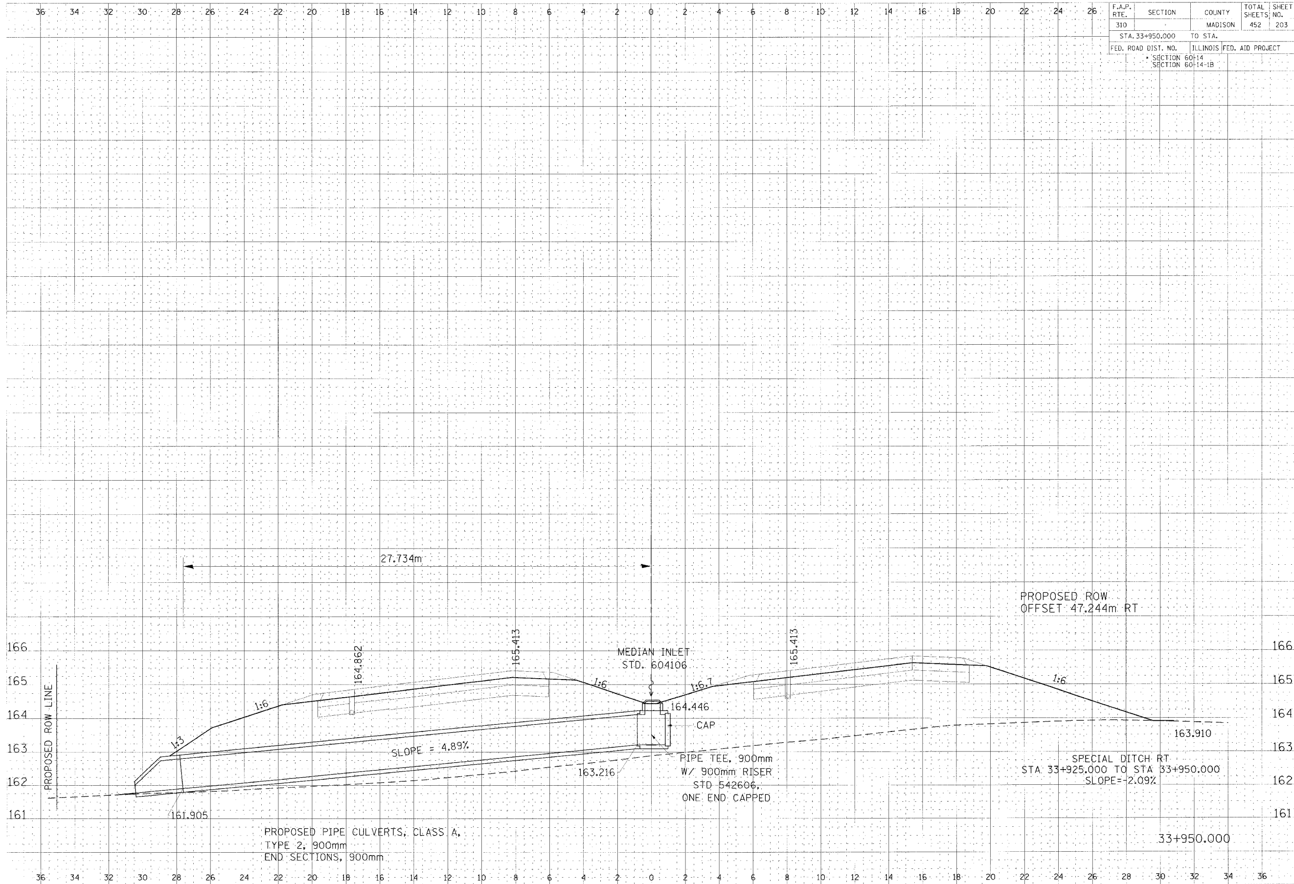
CULVERT PROFILE, FAP ROUTE 310, STA 33+950.000
