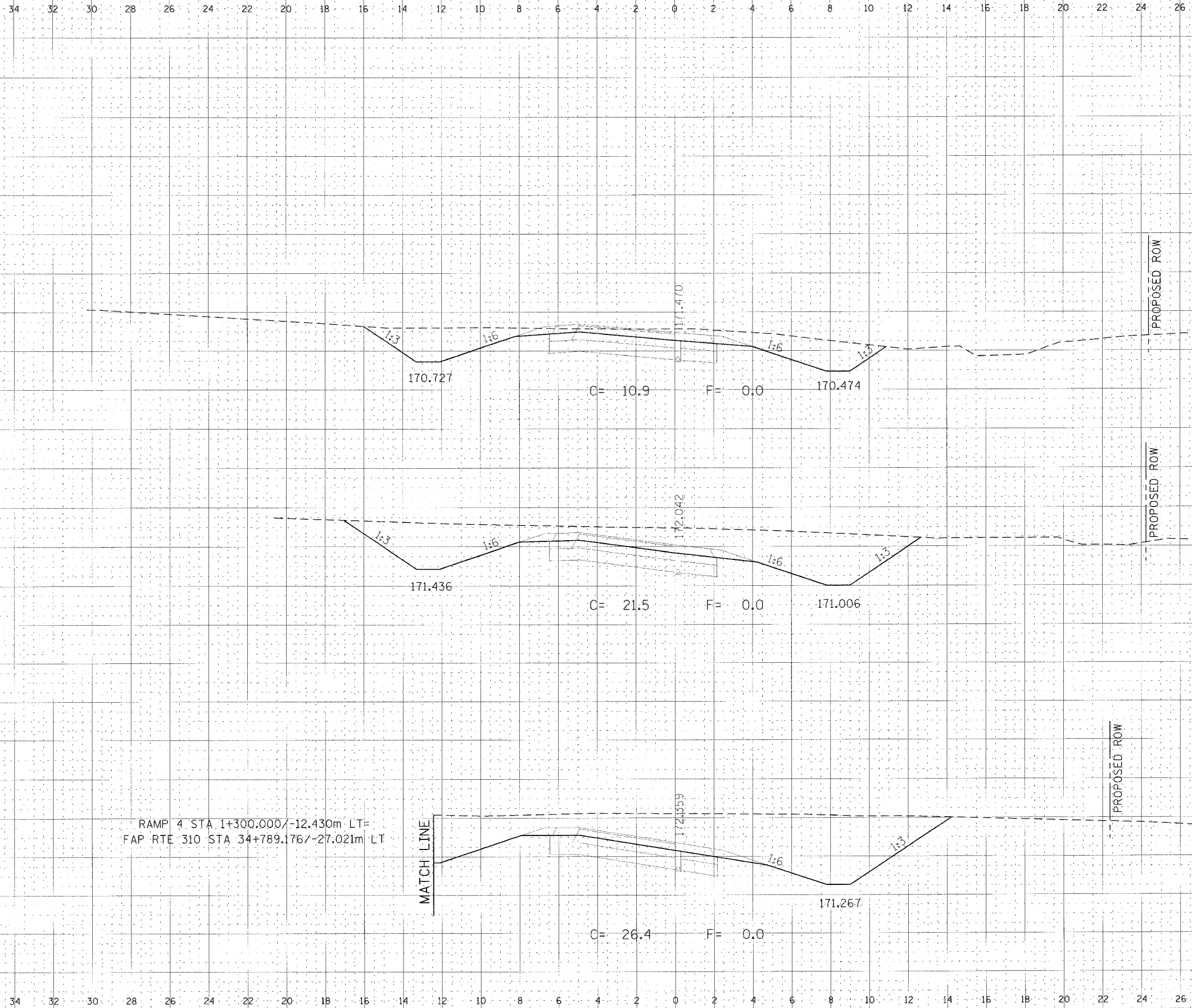
RAMP 4 CROSS SECTION, STA 1+300.000 TO STA 1+350.000
