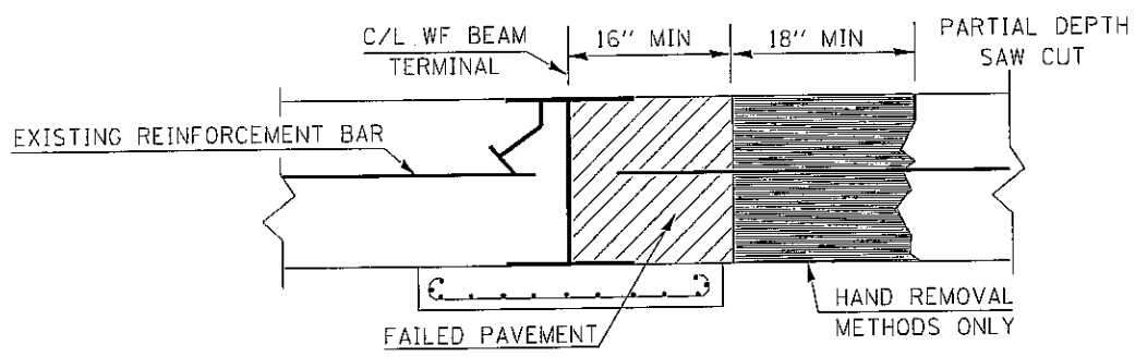
SECTION D-D
