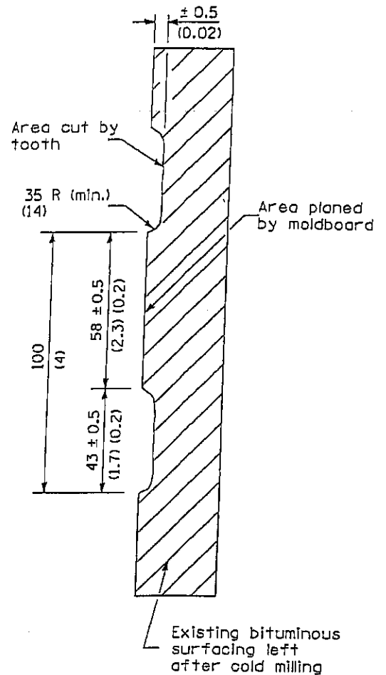
SECTION A-A
