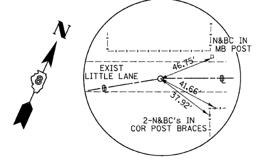
DOMINO LANE PI STA 10+30.31 N - 851255.99 E - 2277627.05 5/8" I. ROD W/CAP
