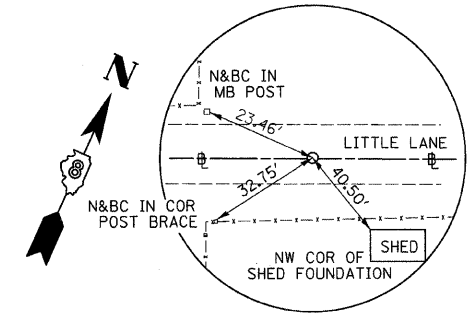
DOMINO LANE POT STA 10+98.05 N - 851273.89 E - 2277693.15 5/8" I. ROD W/CAP
