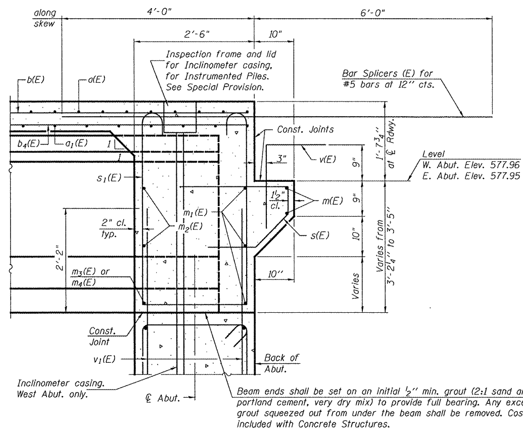
SECTION A-A
