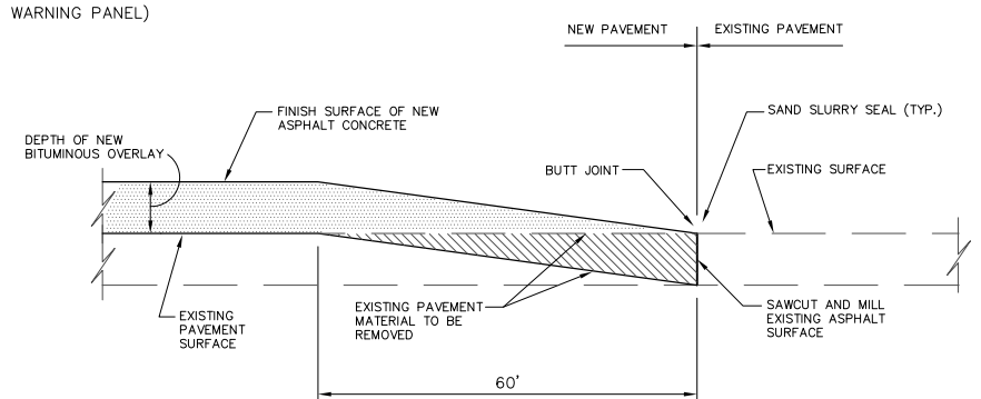
BUTT-JOINT DETAIL N.T.S.
