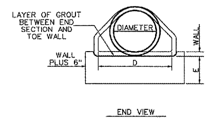
PRECAST CONCRETE FLARED END SECTION N.T.S.
