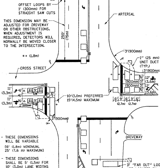
DETAIL 2 N.T.S.
