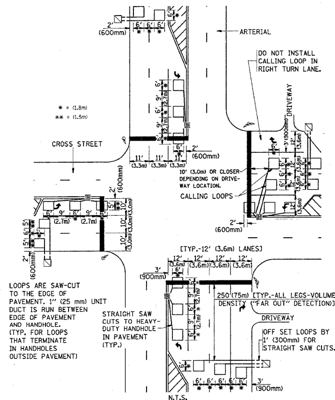
DETAIL 1 N.T.S.
