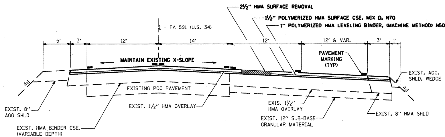
FAP 591 - U.S. RTE. 34 STA. 358+24 to STA. 361+04
