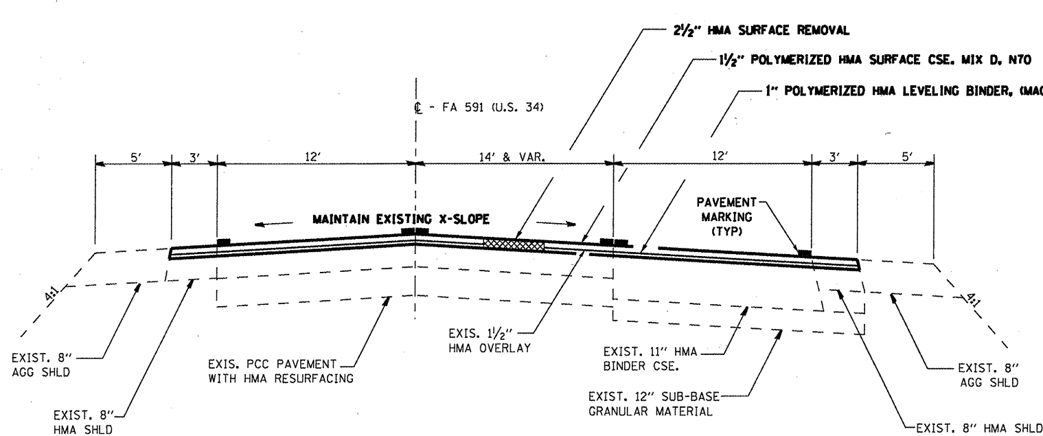
FAP 591 - U.S. RTE. 34 STA. 351+58 to STA. 358+24
