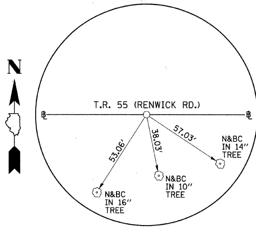
P.O.T. STA. 119+00.00 T.R. 55 (RENWICK RD.) N. 9976.200, E. 6936.716 (5/8" I-ROD)
