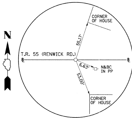
P.O.T. STA. 123+00.00 T.R. 55 (RENWICK RD.) N. 9972.908, E. 7336.703 (5/8" I-ROD)
