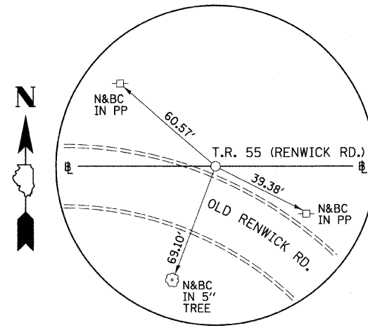
P.O.T. STA. 110+00.00 T.R. 55 (RENWICK RD.) N. 9983.607, E. 6036.747 (5/8" I-ROD)
