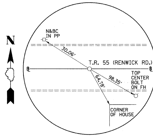
P.O.T. STA. 135+00.00 T.R. 55 (RENWICK RD.) N. 9974.903, E. 8536.673 (MAG NAIL)
