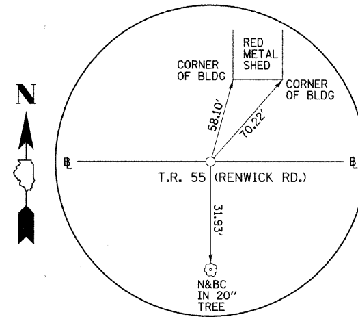
P.O.T. STA. 115+00.00 T.R. 55 (RENWICK RD.) N. 9979.492, E. 6536.780 (5/8" I-ROD)
