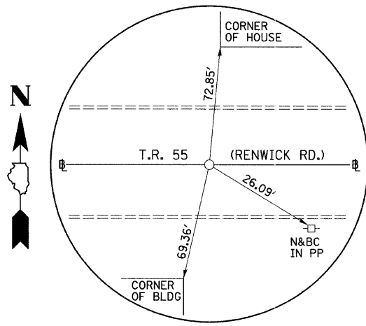
P.O.T. STA. 130+00.00 T.R. 55 (RENWICK RD.) N. 9971.688, E. 8036.683 (MAG NAIL)
