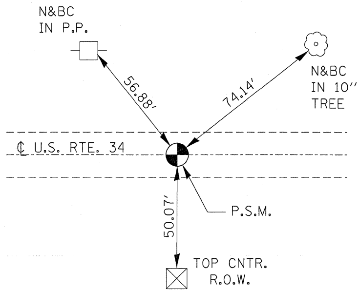
P.I. STA. 40 + 05.37
