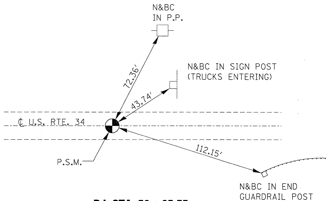
P.I. STA. 52 + 05.75
