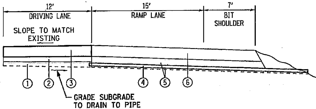
DETAIL A-A
