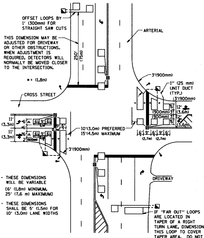
DETAIL 2 N.T.S.
