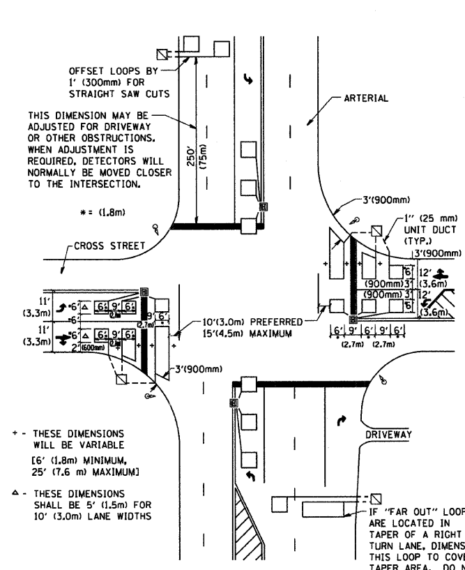
DETAIL 2 N.T.S.
