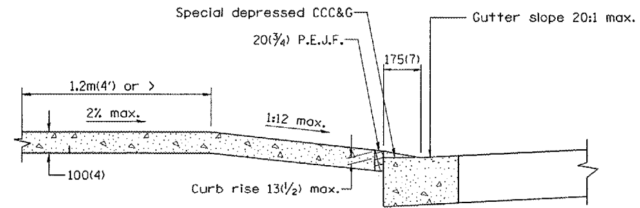
SEC. A-A
