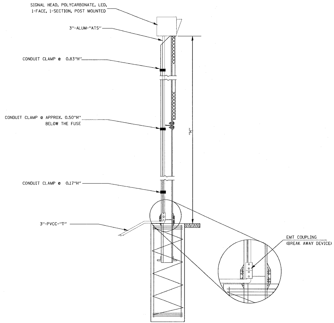
SECTION D-D
