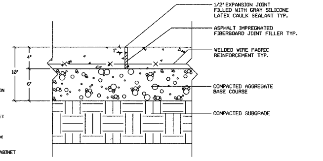
A6 CONCRETE PAVING DETAIL SECTION - N.T.S.
