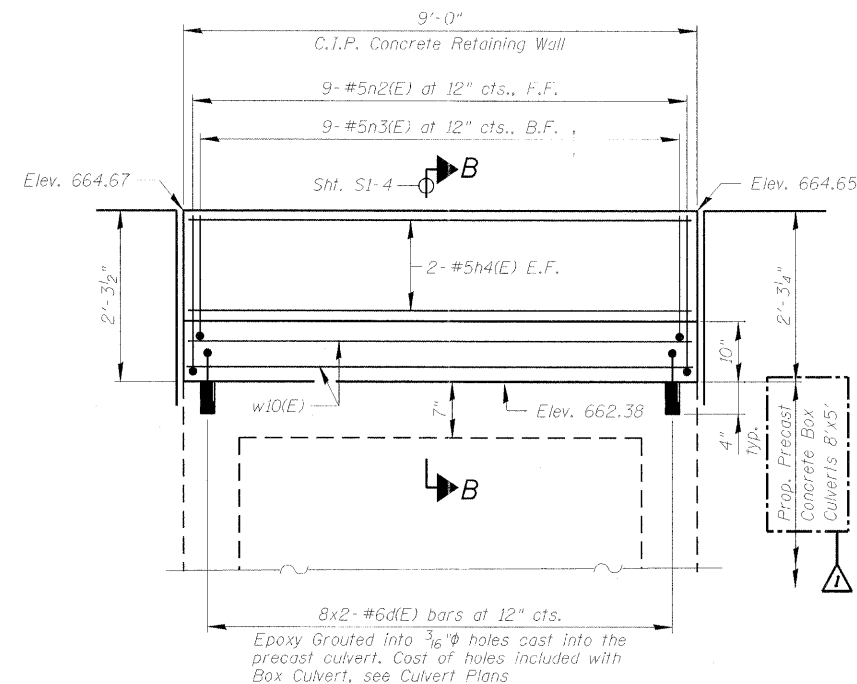
ELEVATION C-C
