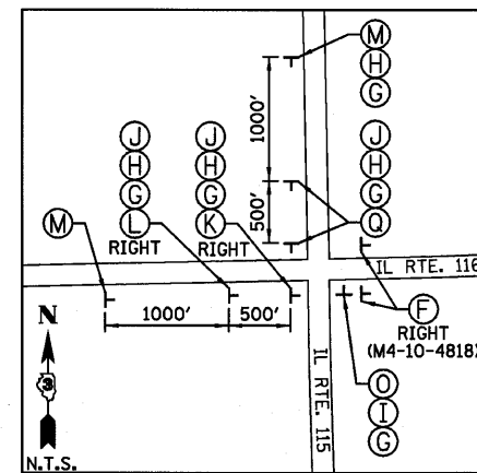
IL RTE. 116 & IL RTE. 115 INTERSECTION (DETAIL "A")
