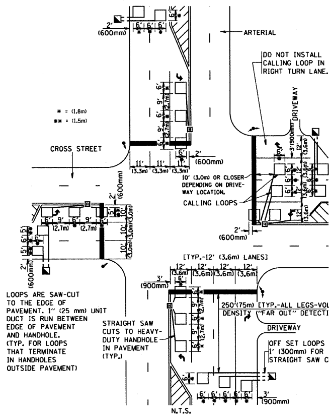
DETAIL 1 N.T.S.
