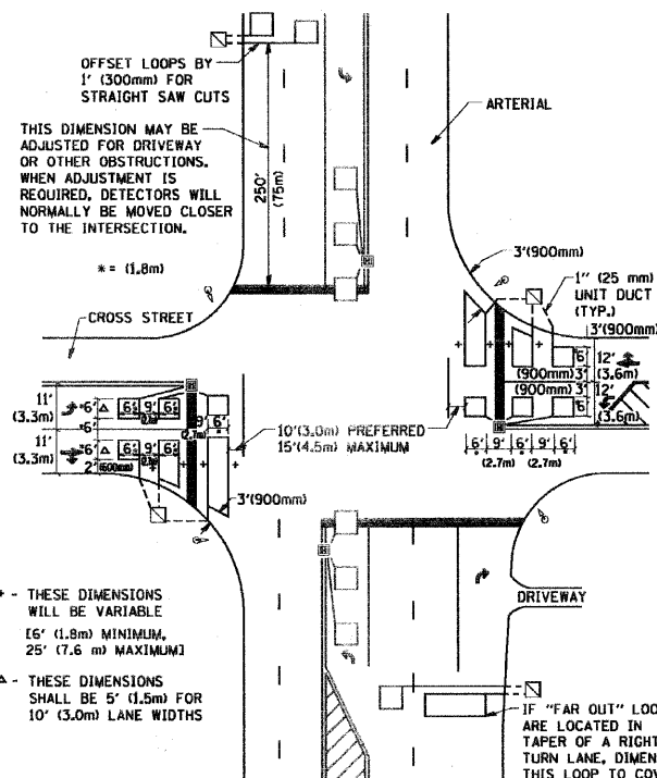
DETAIL 2 N.T.S.
