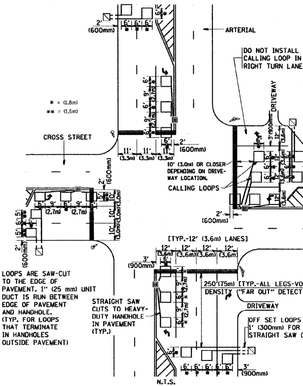
DETAIL 1 N.T.S.
