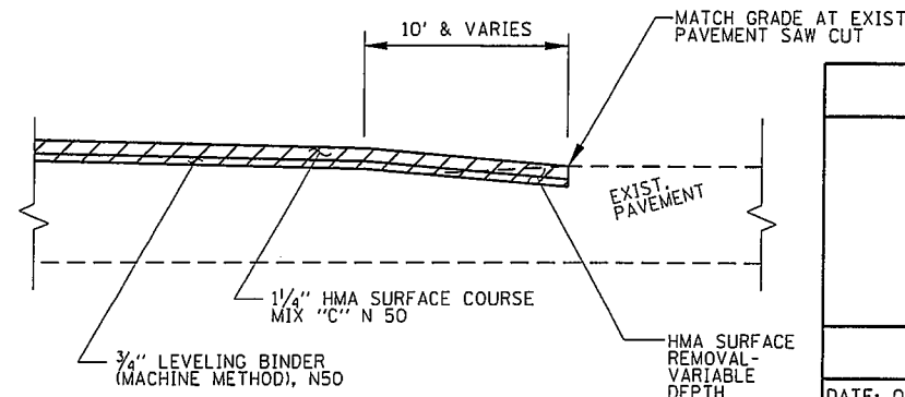
BUTT-JOINT DETAIL
