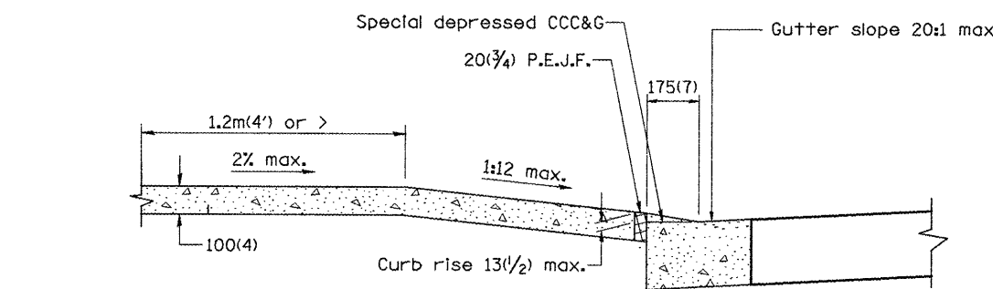
SEC. A-A
