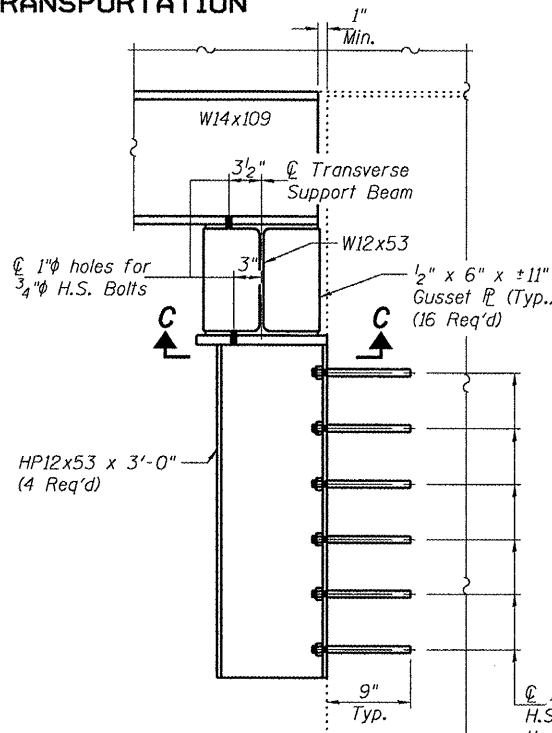
SECTION A-A
