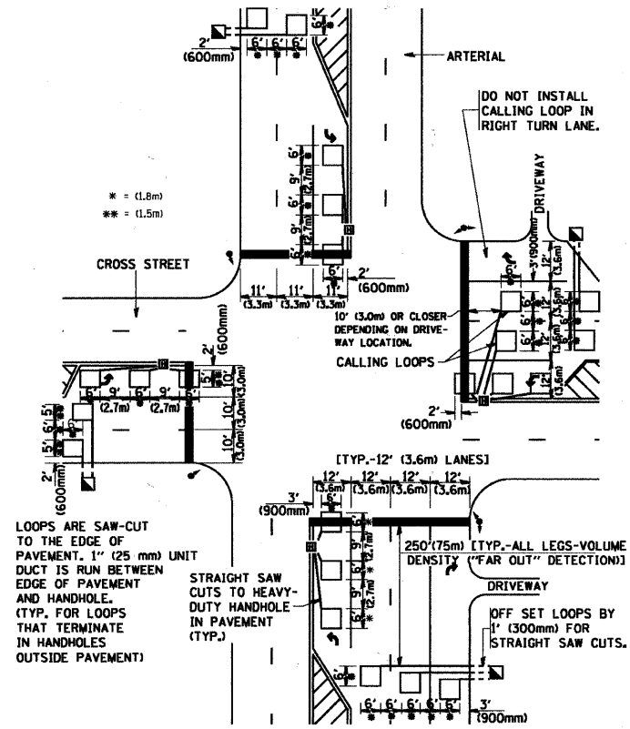
DETAIL 1 N.T.S.
