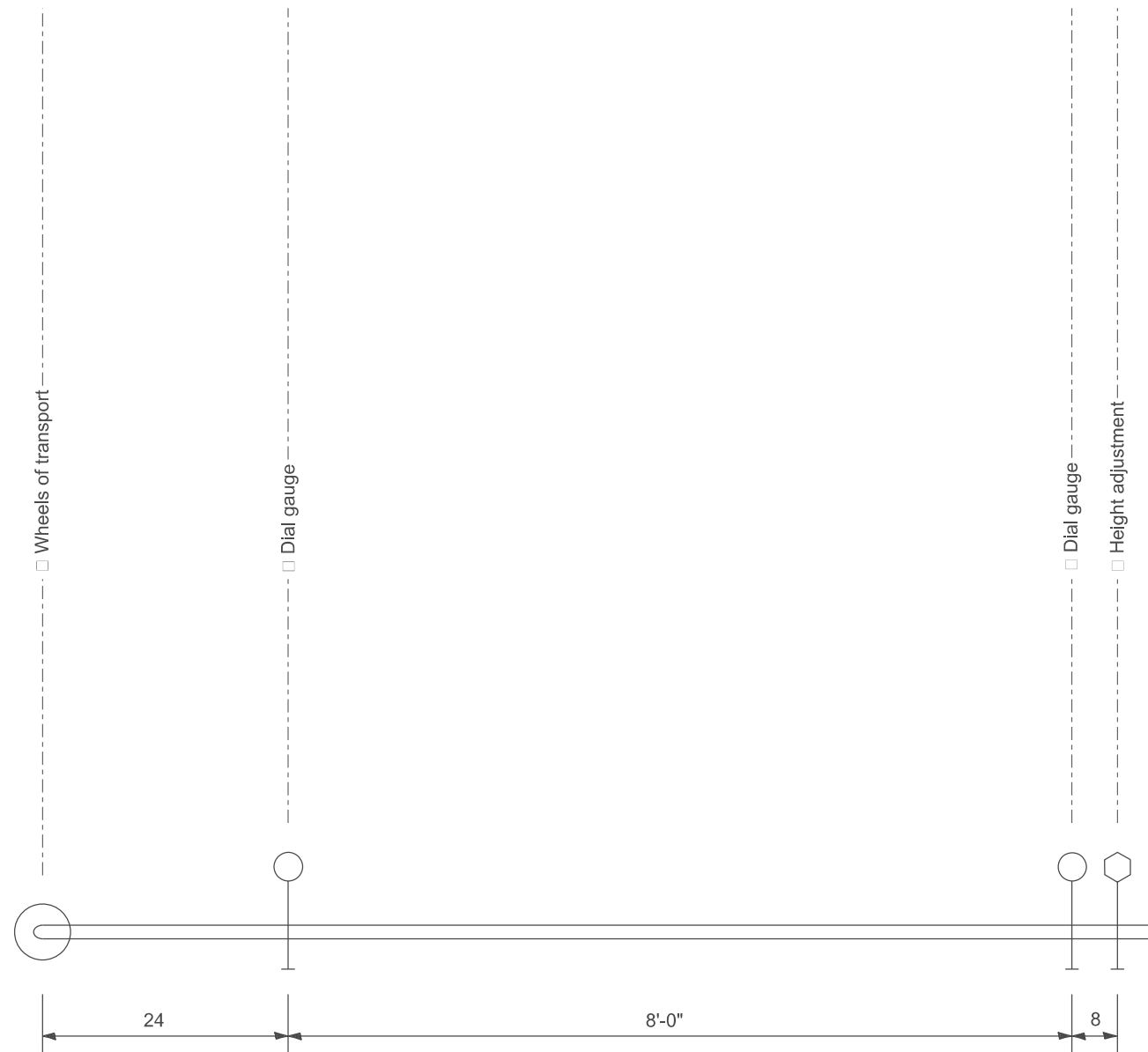
ELEVATION
