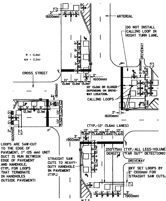
DETAIL 1 N.T.S.
