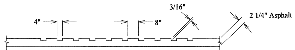
SECTION A-A
