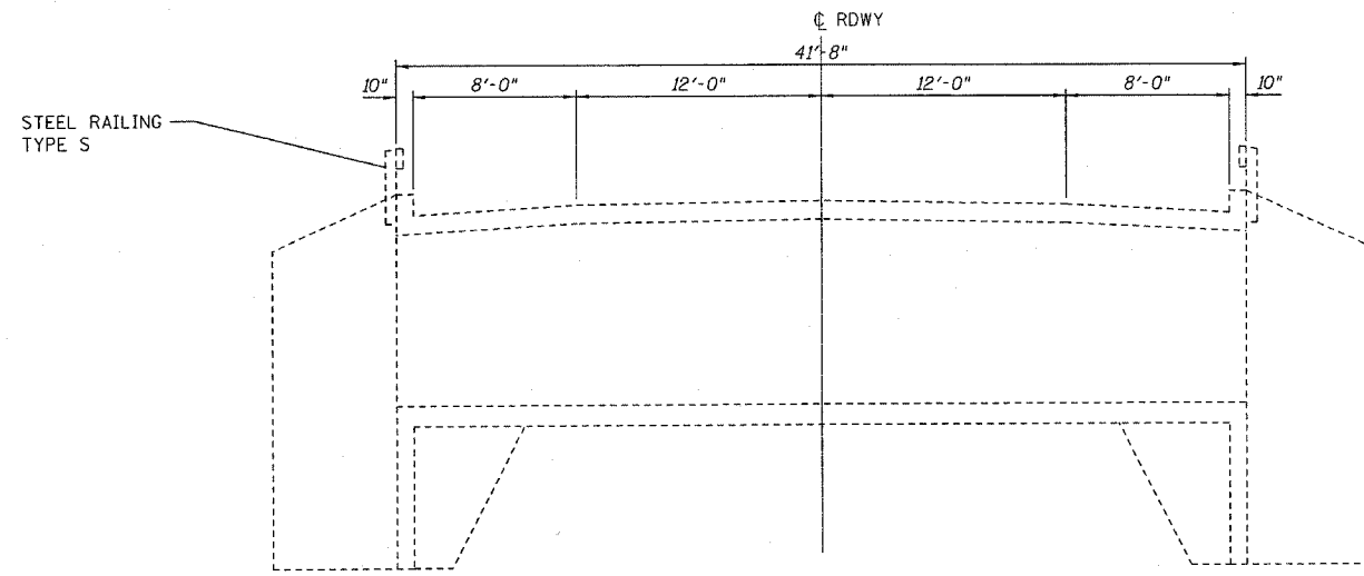
LONGITUDINAL SECTION
