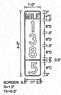
EB-TS-08 STA. 740+20
