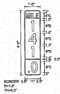
EB-TS-34 STA. 872+50
