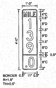
EB-TS-15 STA. 768+10
