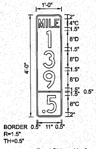
EB-TS-19 STA. 794+50
