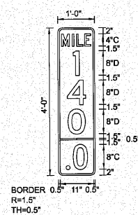
EB-PM-25 STA. 823+70
