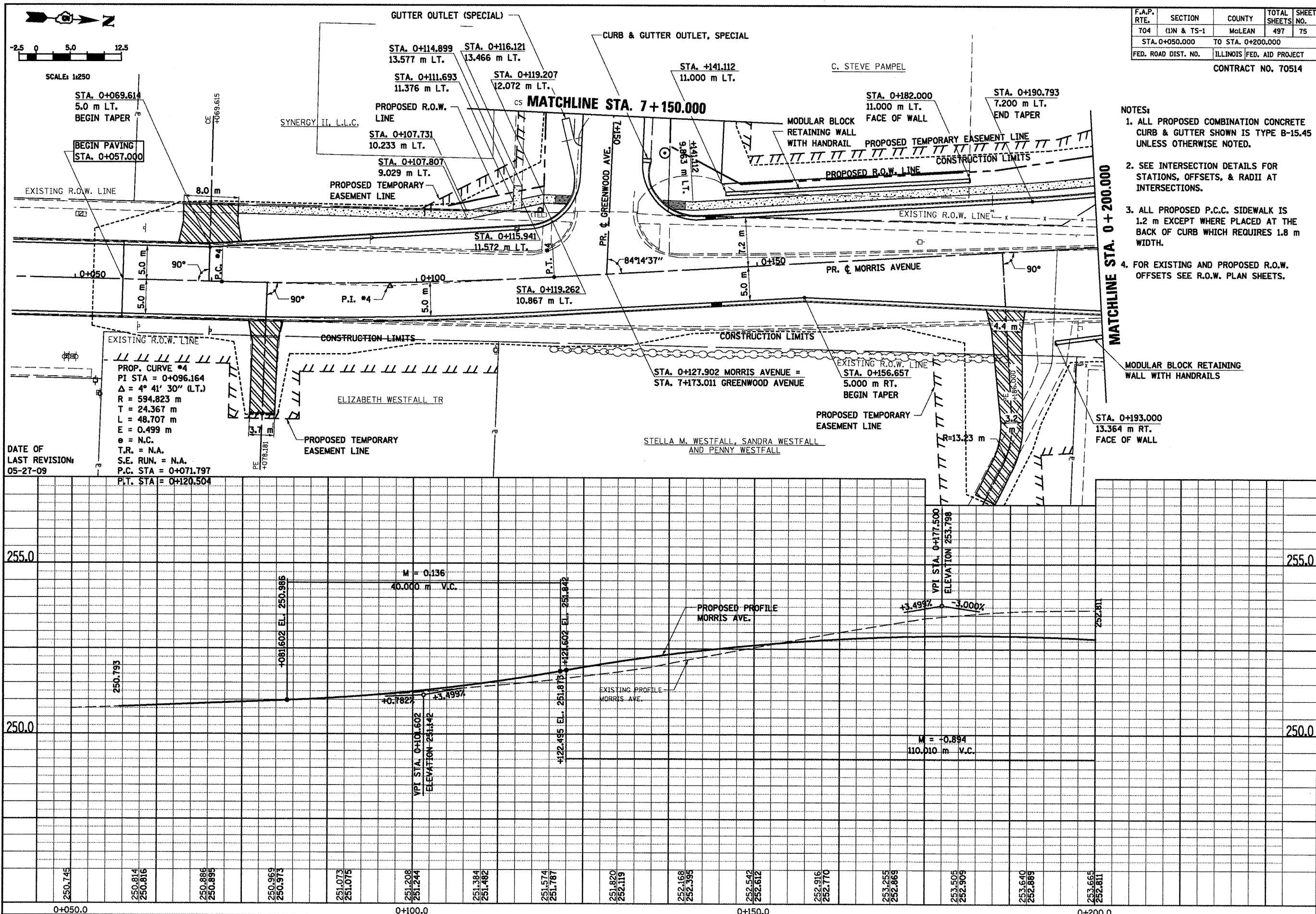
MORRIS AVENUE, PLAN & PROFILE, STA. 0+050.000 TO STA. 0+200.000
