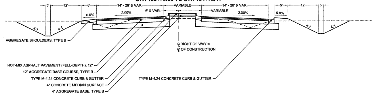
AUBURN ROAD STA 93+27.99 TO STA 99+30.00 STA 100+70.00 TO STA 104+75.41
