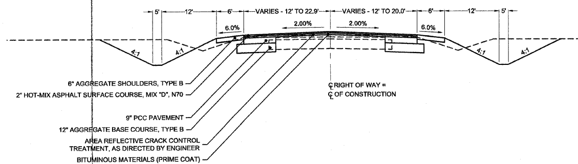
AUBURN ROAD STA 104+75.41 TO STA 110+76.45
