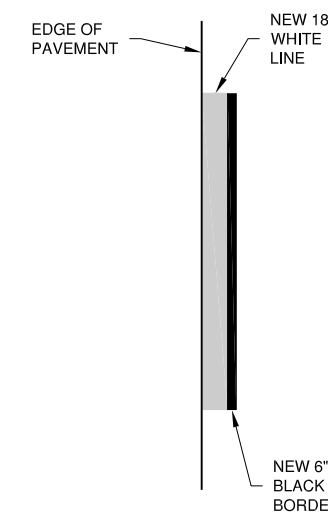
3 RUNWAY 18/36 EDGE STRIPE CONTINUOUS N.T.S.
