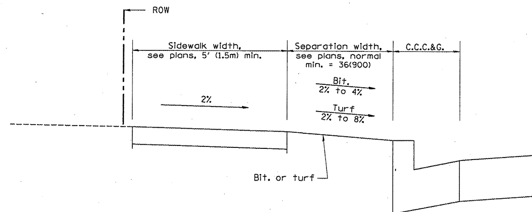
SECTION D-D
